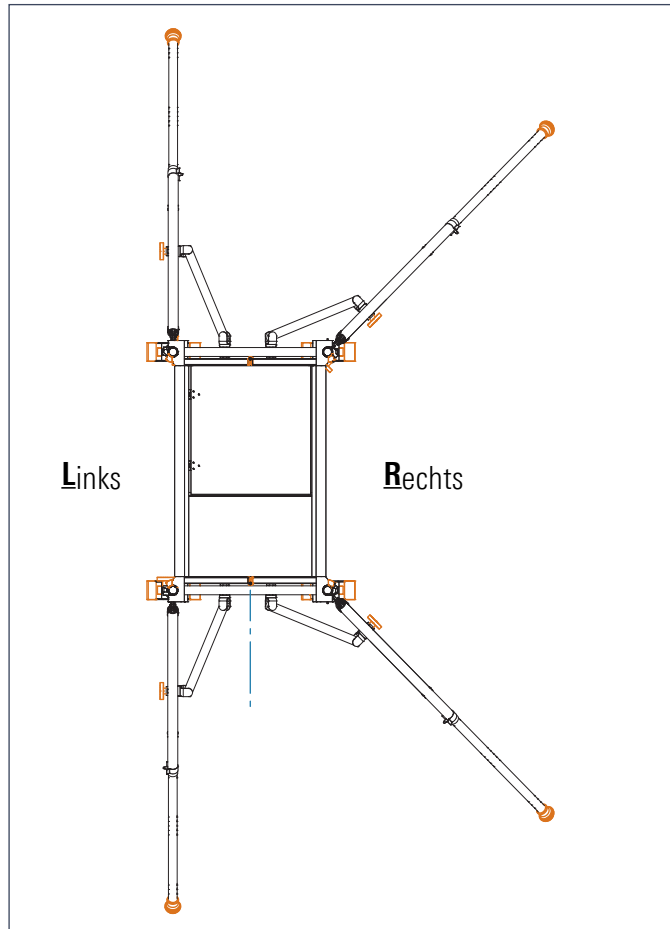
Aufbau seitlich:
