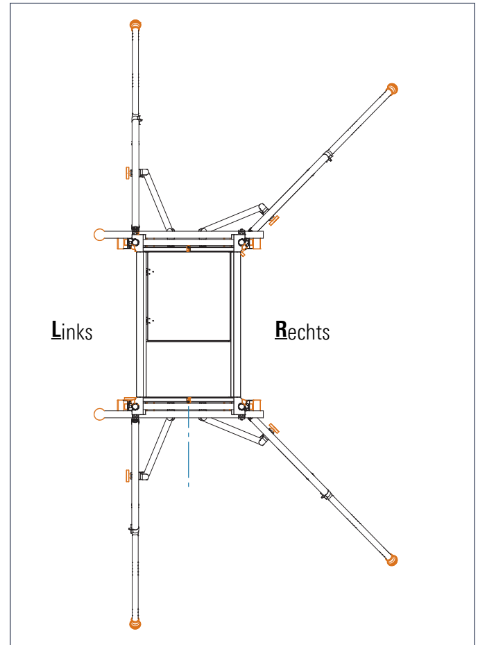
Aufbau Wandabstützung:
